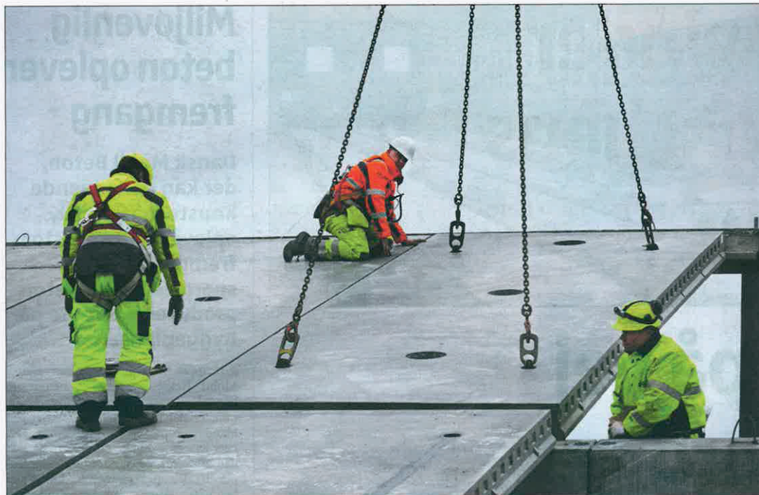
Montering af Abeos betondæk på Gammel Hellerup Gymnasium.
